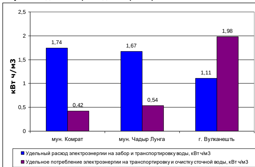
Рисунок 6: Удельный расход электроэнергии в системах ВСиВО в городах, кВт/м 3
